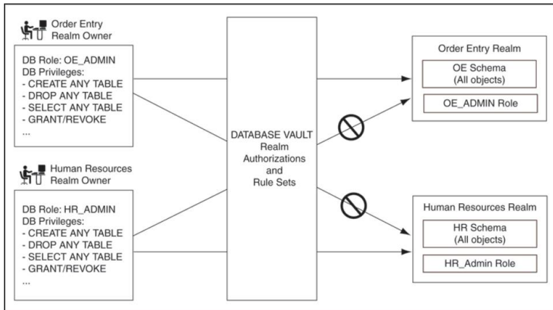
Figura 1 - Funcionamento de autorizações para Realms e donos de Realms [HUEY et al., 2008]
